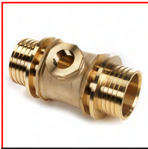
T-stuk met binnendraad
